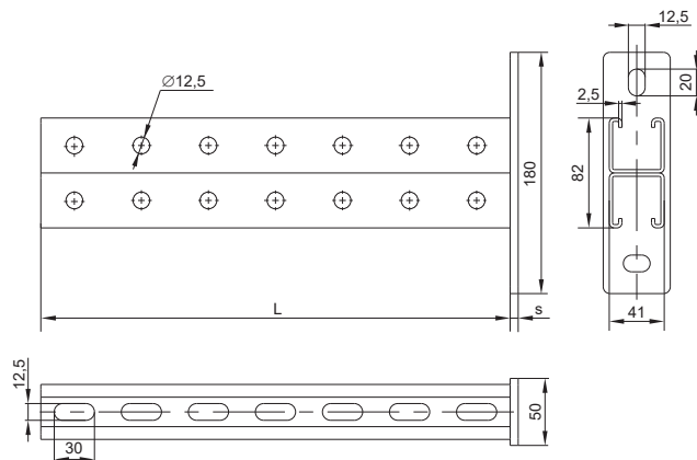
Рисунок / Figure / Сурет 5 – Консоль двойная / Double console / Қосарлы консолі STRUT 41×41
