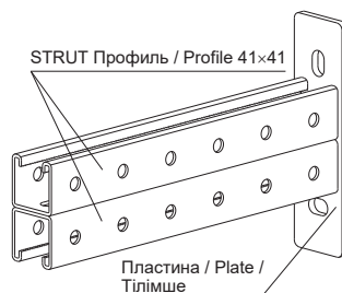
Консоль двойная / Double console / Қосарлы консолі STRUT 41×41
