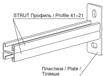
Консоль двойная / Double console / Қосарлы консолі STRUT 41×21
