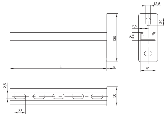
Рисунок / Figure / Сурет 2 – Консоль / Console / Консолі STRUT 41×21
