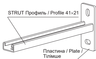
Консоль / Console / Консолі STRUT 41×21
