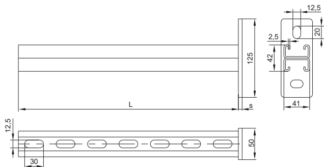
Рисунок / Figure / Сурет 4 – Консоль двойная / Double console / Қосарлы консолі STRUT 41×41
