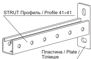
Консоль / Console / Консолі STRUT 41×41
