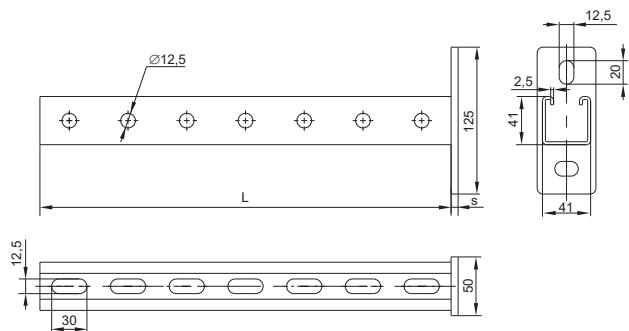
Рисунок / Figure / Сурет 3 – Консоль / Console / Консолі STRUT 41×41
