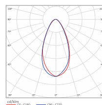
Угол излучения 60°
