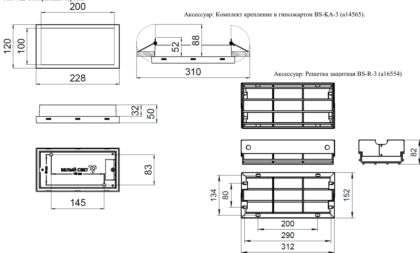
Рис. №2 Габаритный чертёж.
