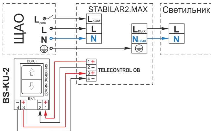
Рис 5. Пример схемы подключения Кнопки управления BS-KU-2 или BS-KU-4
