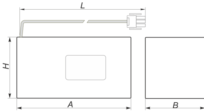
Рис. 6 Батарея BS-2P4S-IFpR-H-32/70- 6,0/2F-HB300-MATE/N/LOK/3N-1 а27901
