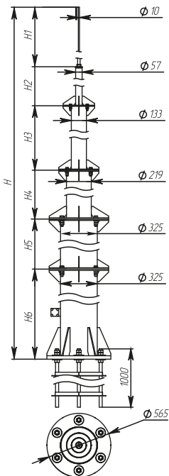
Рисунок / Figure / Сурет 14 – Мачты высотой 27000, 28500, 30000 мм / Air-termination mast 27000, 28500, 30000 mm high / Биіктігі 27000, 28500, 30000 мм діңгектер
