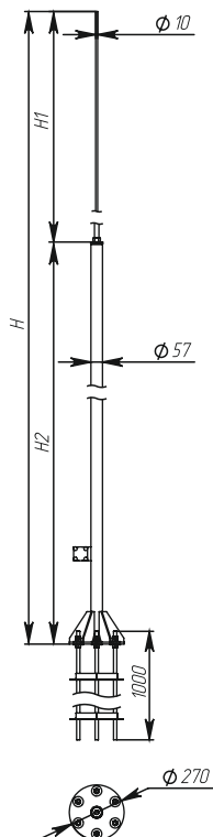
Рисунок / Figure / Сурет 1 – Мачты высотой 6000, 7500 мм / Air-termination mast 6000, 7500 mm high / Биіктігі 6000, 7500 мм діңгектер
