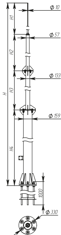
Рисунок / Figure / Сурет 7 – Мачта высотой 16500 мм / Air-termination mast 16500 mm high / Биіктірі 16500 мм діңгек
