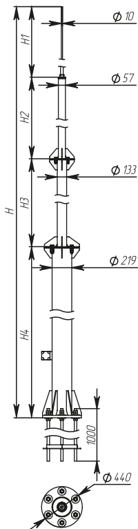
Рисунок / Figure / Сурет 8 – Мачта высотой 18000 мм / Air-termination mast 18000 mm high / Биіктірі 18000 мм діңгек
