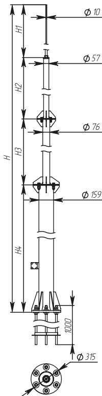
Рисунок / Figure / Сурет 5 – Мачта высотой 13500 мм / Air-termination mast 13500 mm high / Биіктірі 13500 мм діңгек
