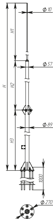
Рисунок / Figure / Сурет 3 – Мачта высотой 10500 мм / Air-termination mast 10500 mm high / Биіктігі 10500 мм діңгек
