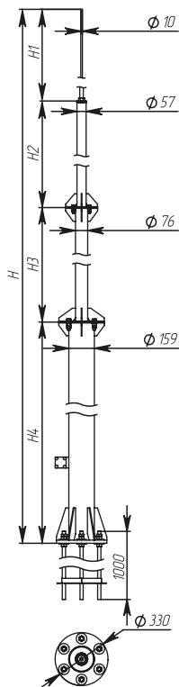
Рисунок / Figure / Сурет 6 – Мачта высотой 15000 мм / Air-termination mast 15000 mm high / Биіктірі 15000 мм діңгек
