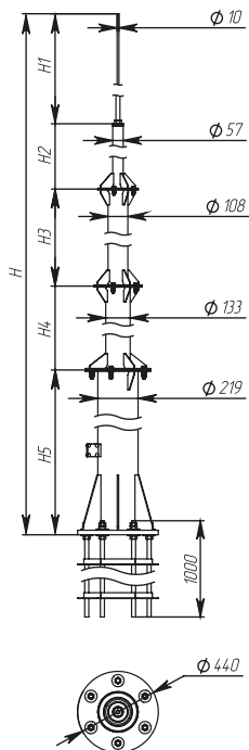
Рисунок / Figure / Сурет 9 – Мачта высотой 19500 мм / Air-termination mast 19500 mm high / Биіктірі 19500 мм діңгек
