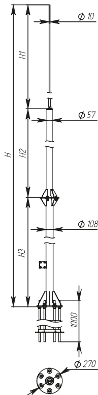
Рисунок / Figure / Сурет 4 – Мачта высотой 12000 мм / Air-termination mast 12000 mm high / Биіктірі 12000 мм діңгек
