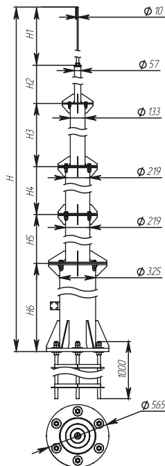
Рисунок / Figure / Сурет 13 – Мачта высотой 25500 мм / Air-termination mast 25500 mm high / Биіктігі 25500 мм діңгек
