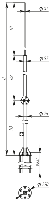
Рисунок / Figure / Сурет 2 – Мачта высотой 9000 мм / Air-termination mast 9000 mm high / Биіктігі 9000 мм діңгек
