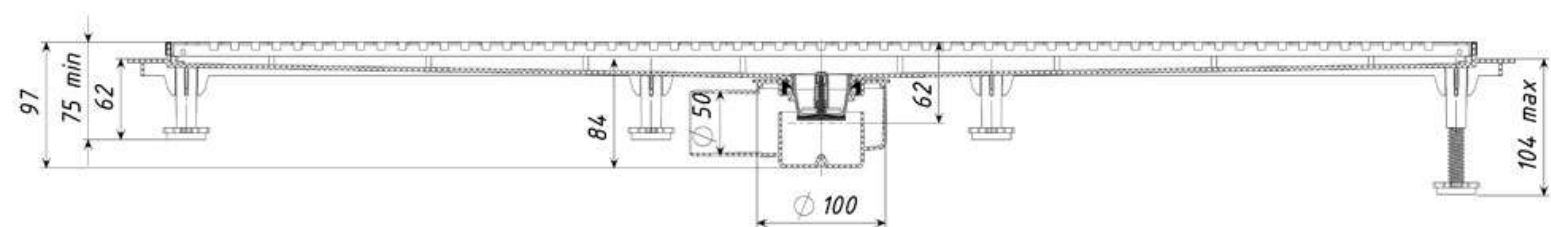
Вариант установки механического "сухого" затвора
