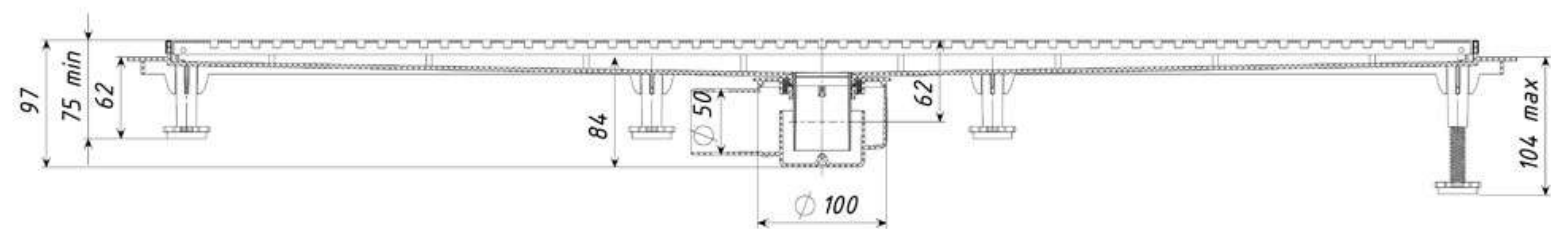
Вариант установки с гидрозатвором
