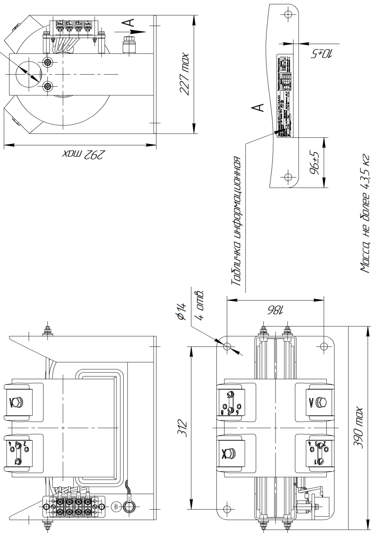
Рисунок А.6 – Габаритные, установочные, присоединительные размеры и масса трансформаторов ОЛС-НТЗ-2.5/6(10)
