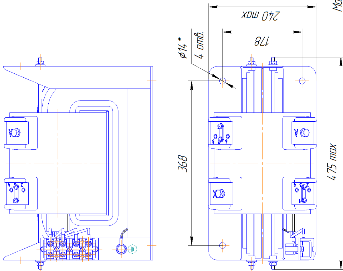
Рисунок А.7 – Габаритные, установочные, присоединительные размеры и масса трансформаторов ОЛС-НТЗ-5.0/6(10)
