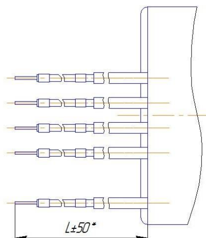
Рисунок А.8 – Исполнение вторичных выводов трансформаторов ОЛС(П)-НТЗ-0.63/6(10)
