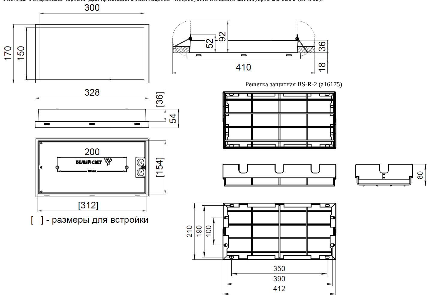
Рис. №2 Габаритный чертёж. Для крепления в гипсокартон потребуется комплект аксессуаров BS-КА-3 (a14565).
