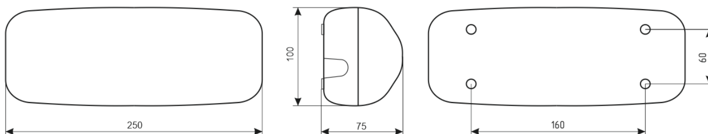
Рис. №3 Габаритный чертёж.
