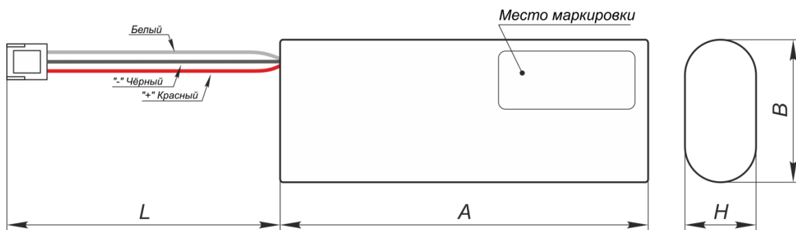
Характеристики АКБ
