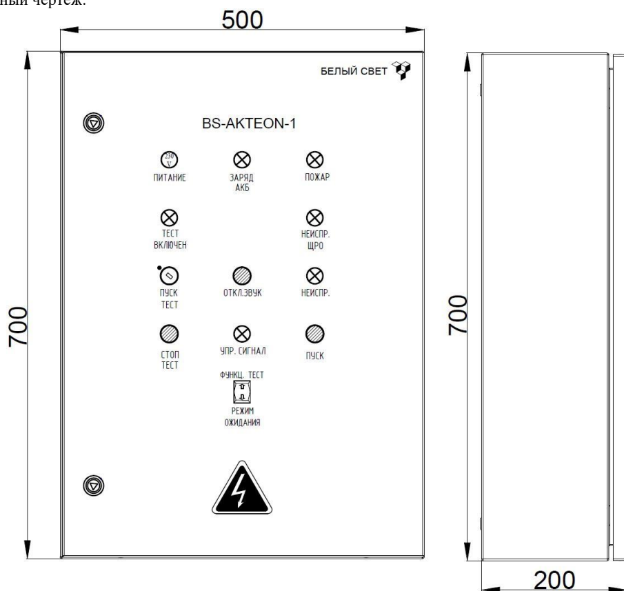
Рис. №2 Установочный чертёж.
