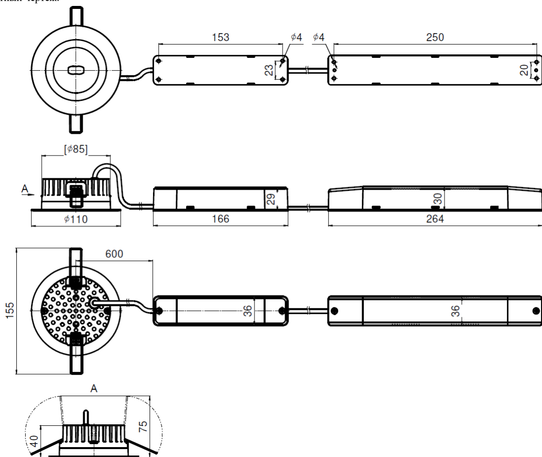
Рис. №2 Габаритный чертёж.
