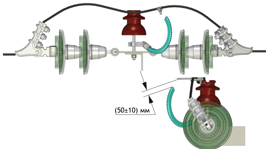
Рисунок 15 - Эскиз установки разрядника совместно с натяжной стеклянной изоляцией на анкерной опоре и зажима на проводе, в случае закрепления шлейфа на штыревом изоляторе
