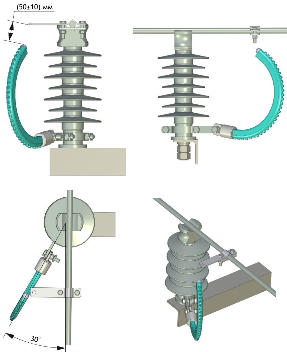
Рисунок 13 - Эскиз установки разрядника совместно с опорной изоляцией и зажима на проводе
