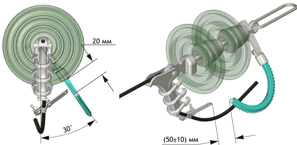
Рисунок 14 - Эскиз установки разрядника совместно с натяжной стеклянной изоляцией и зажима на проводе
