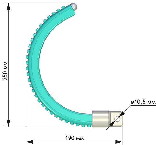
Рисунок 2 - Внешний вид, габаритные, установочные и присоединительные размеры разрядного элемента разрядника
