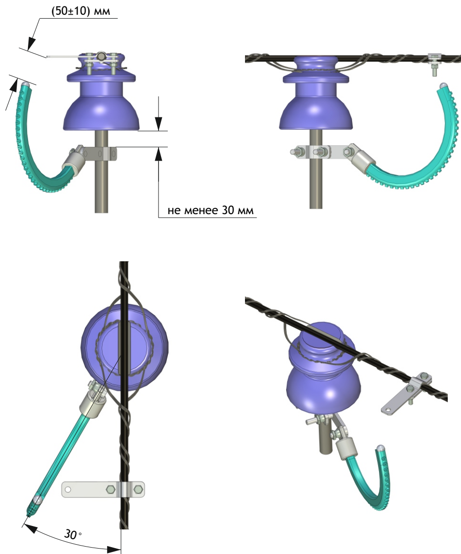
Рисунок 11 - Эскиз установки разрядника совместно со штыревой изоляцией и зажима на проводе
