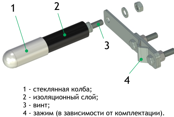
Рисунок 7 - Зажим с электродом-индикатором
