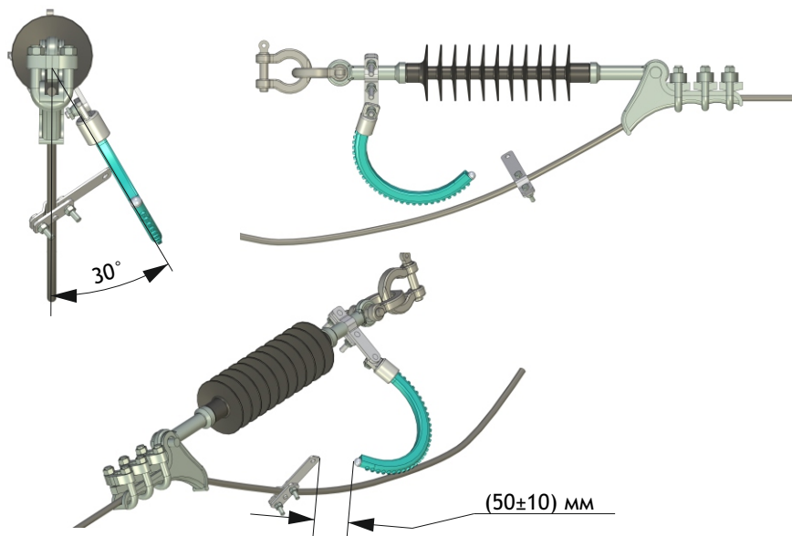
Рисунок 16 - Эскиз установки разрядника совместно с натяжной полимерной изоляцией и зажима на проводе
