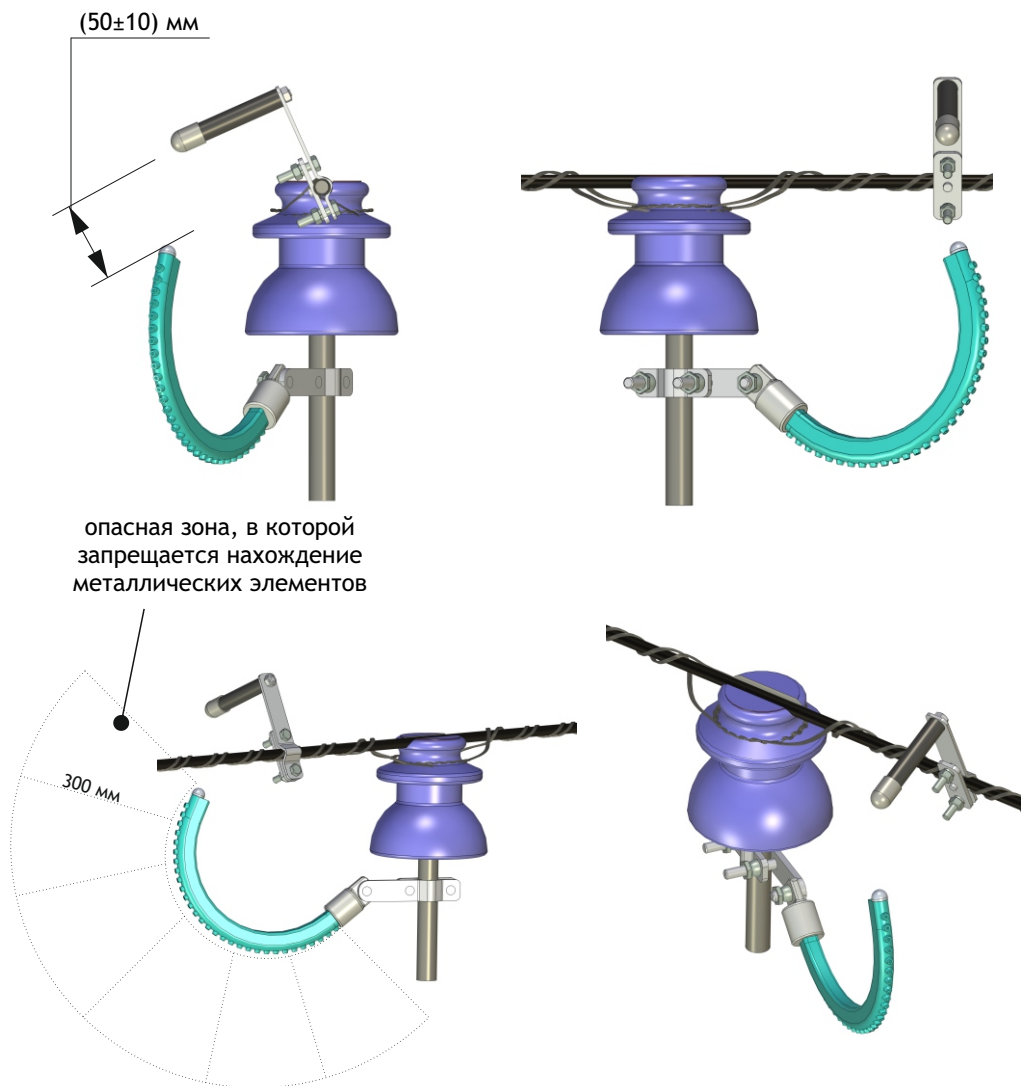
Рисунок 12 - Эскиз установки разрядника совместно со штыревой изоляцией и зажима на провод, снабженного электродом-индикатором
