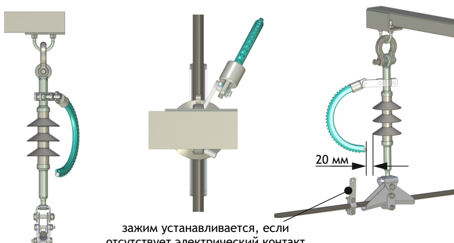
Рисунок 17 - Эскиз установки разрядника совместно с подвесной полимерной изоляцией
