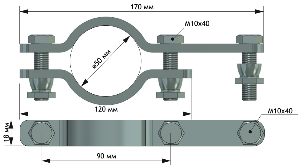
Рисунок 4 - Внешний вид, габаритные, установочные и присоединительные размеры кронштейна для установки разрядника совместно с опорной изоляцией
