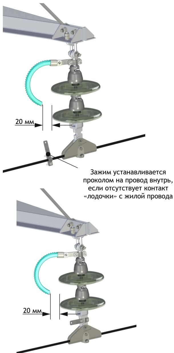
Рисунок 18 - Эскиз установки разрядника совместно с подвесной стеклянной изоляцией
