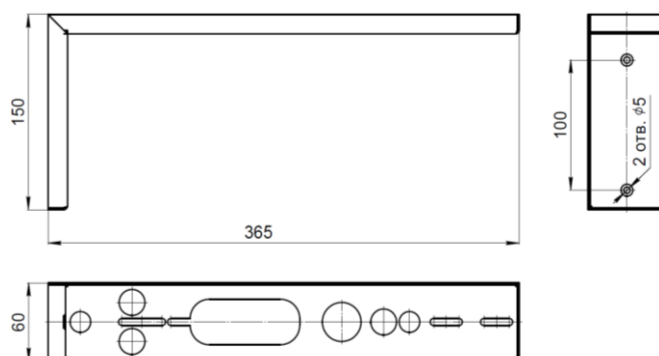
Рис. 3.2 Кронштейн BS-K-3
