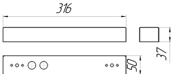
Рис.3.1 Крышка BS-KR-3 (Для монтажа на шпильки M8)
