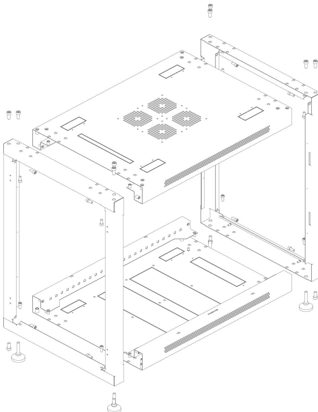
Рисунок 1 – установка основания и крышки.
