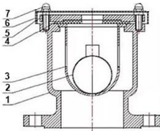
Рисунок 1 - Деталировка
