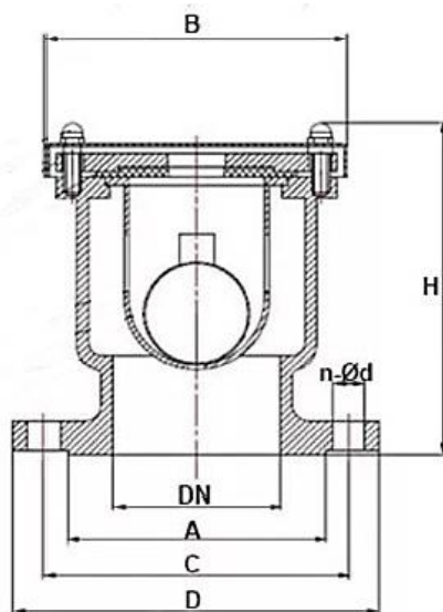
Рисунок 2- Размеры
