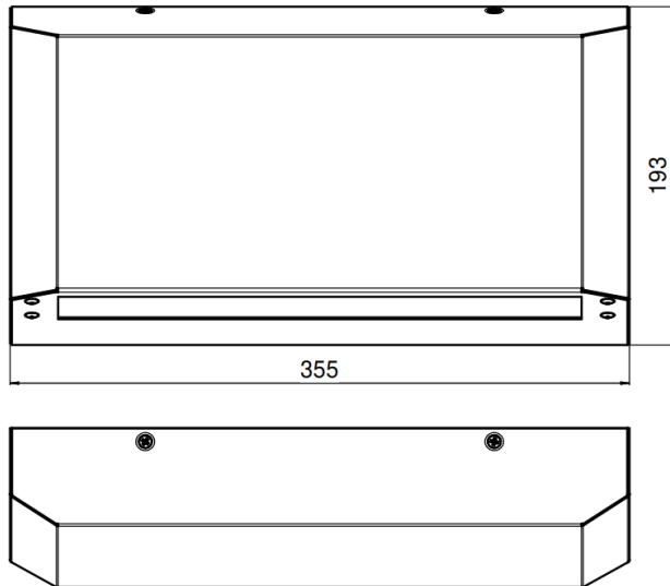
Рис. №2 Габаритный чертёж.
