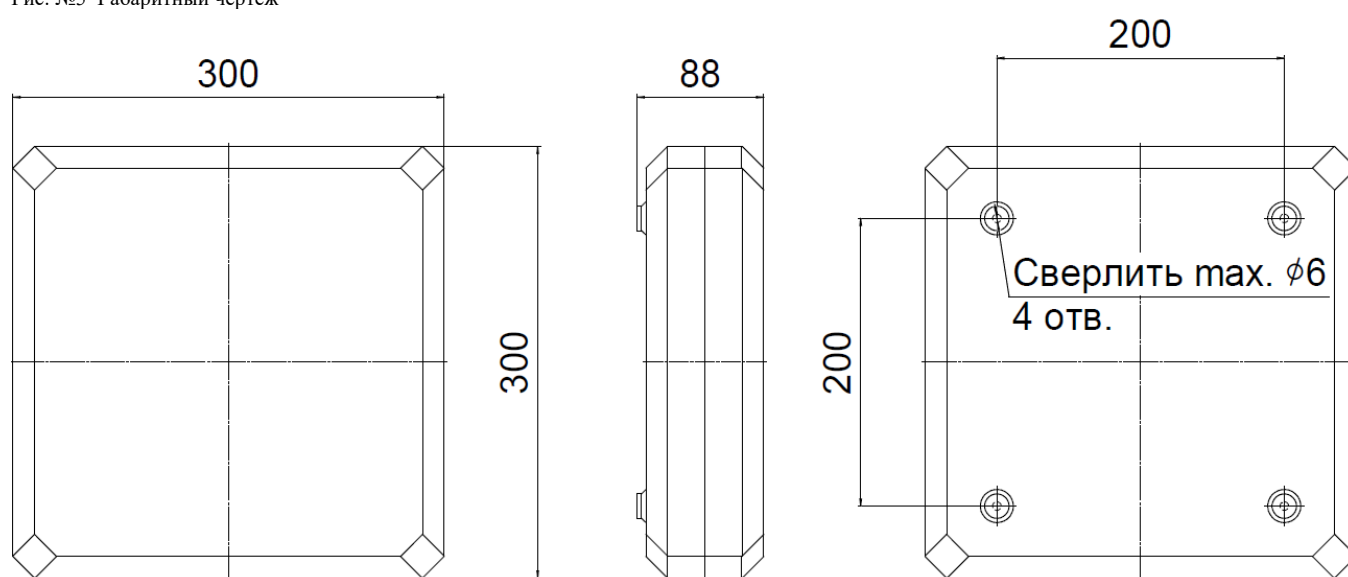
Рис. №5 Габаритный чертёж
