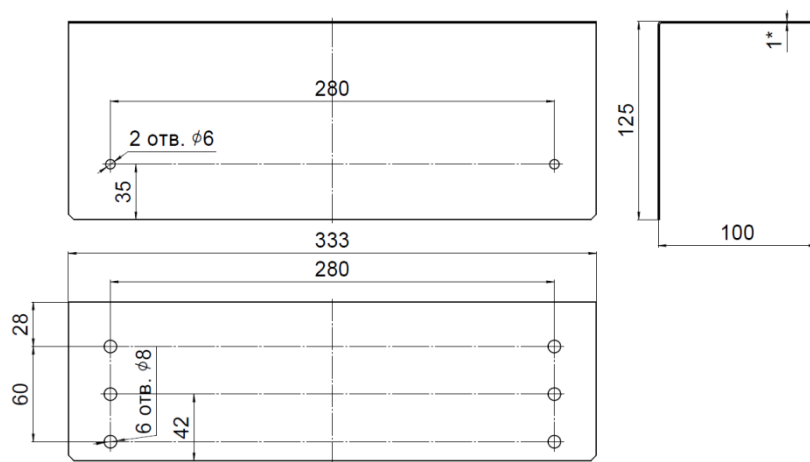
Рис.4 – Аксессуар для крепления к потолку для BS-DBU-53-L2-INEX12 Кронштейн BS-K-30 (a22635)
