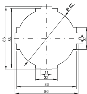
Рисунок 3 – Размеры отверстий под шины и кабели
