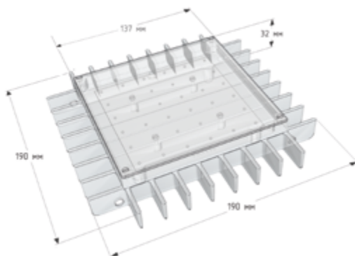
Габаритные размеры
