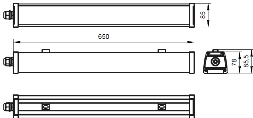
Рис. №2 Габаритный чертёж.
