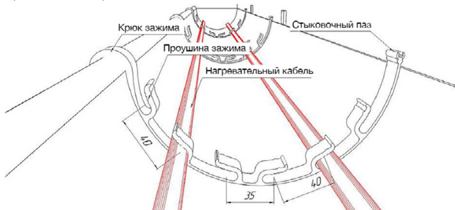
Рис. 3 (Зажим RX/B1-6)
