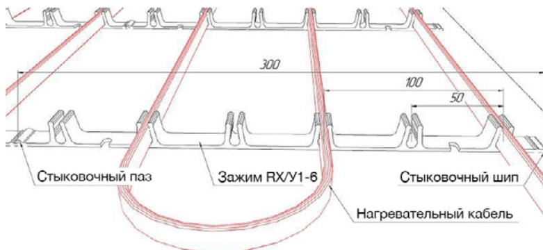
Рис. 5 (Зажим RX/Y 1-6)
