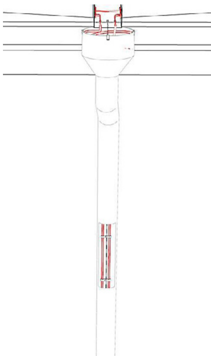
Рис. 4 (Крепление нагревательного кабеля с использованием зажима RX/3T, сливное колено)
