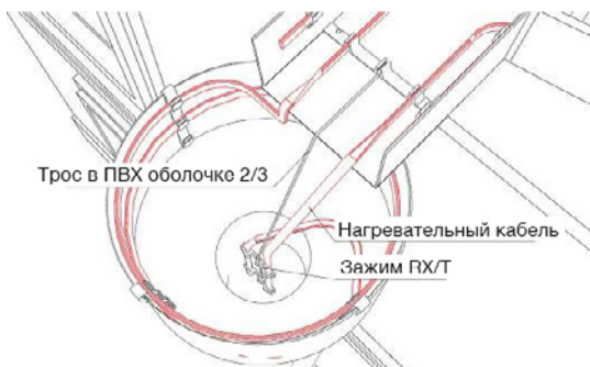
Рис. 3 (Расположение кабеля в трубе)
