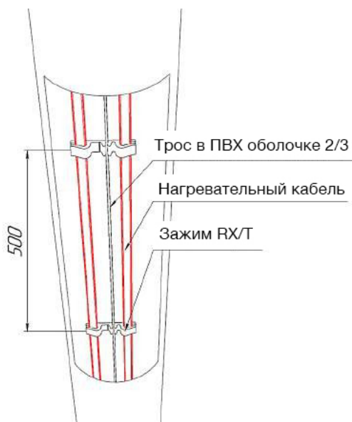
Рис. 5 (Зажим RX/Т)
