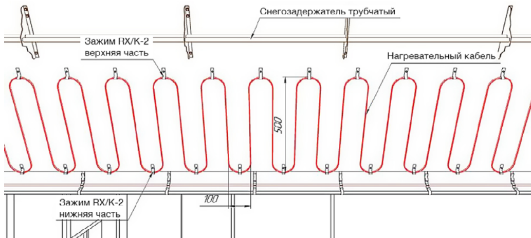
Рис. 2 (Вид сверху)
