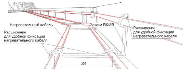
Рис. 3 (Зажим RX/3B)
