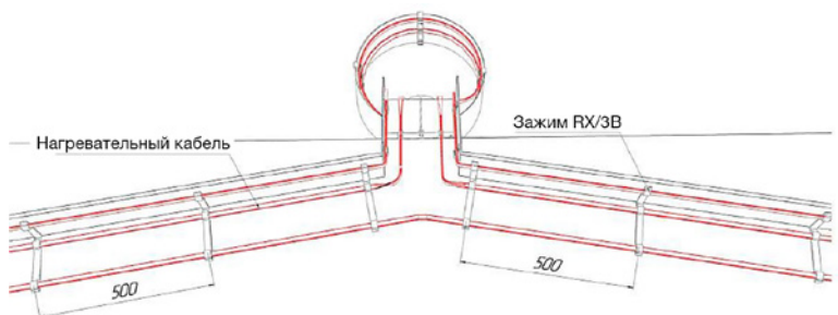
Рис. 2 (Вид сверху)
