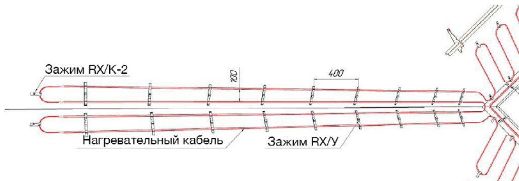
Рис. 2 (Вид сверху)
