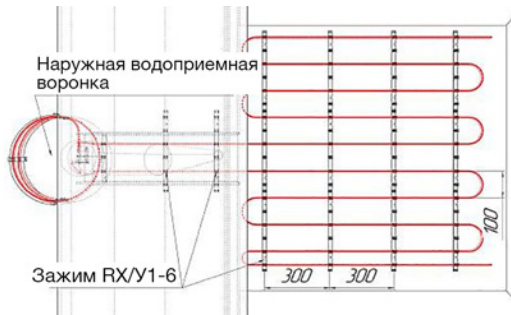
Рис. 5 (Зажим RX/Y 1-6)
