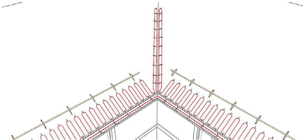
Рис. 2 (Вид сверху)
