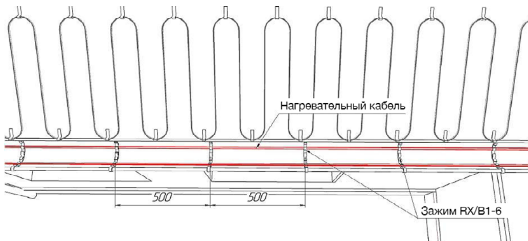
Рис. 3 (Зажим RX/B1-6)
