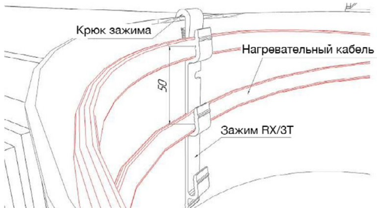
Рис. 3 (Зажим RX/3T)
