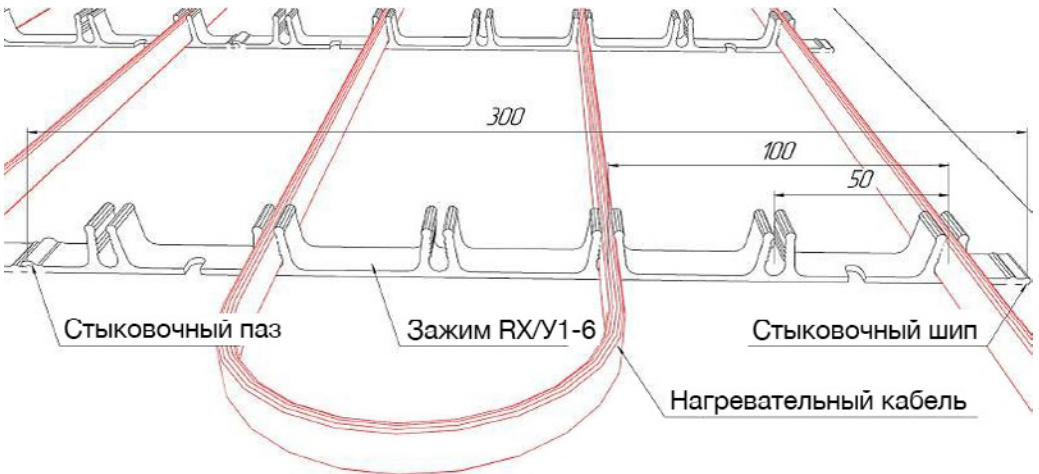
Рис. 5 (Зажим RX/Y 1-6)
