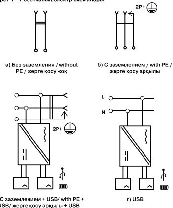
Рисунок 1 – Электрические схемы розетки / Figure 1 – Electrical schematic of socket / Сурет 1 – Розетканың электр схемалары
