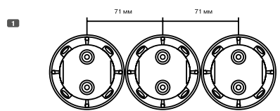
КРАТКОЕ РУКОВОДСТВО ПО МОНТАЖУ РОЗЕТОК Quick installation guide / розеткаларды орнату бойынша қысқаша нұсқаулық Установите подрозетники с шагом 71 мм. Install the mounting box with a distance of 71 mm. / 71 мм қадаммен розеткаларды орнатыңыз.
