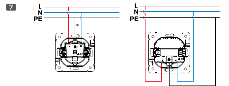
Схема подключения / Connecting scheme / Қосылу схемасы
