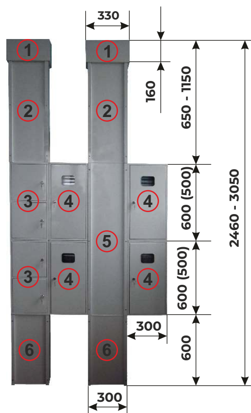
Элементы устройства УЭРМ
