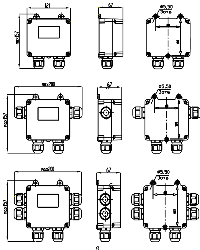
Рис. 1. Установочные и габаритные размеры устройства соединительного.
