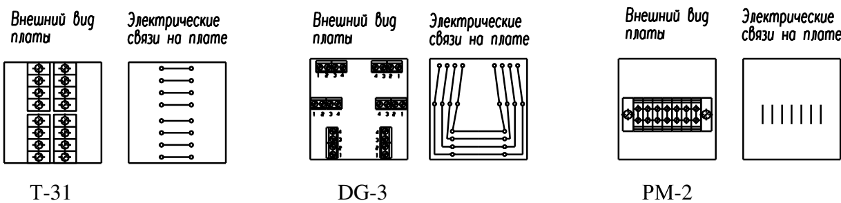
Рис. 3. Электрические связи на плате устройства соединительного УСБ «СЕВЕР»
