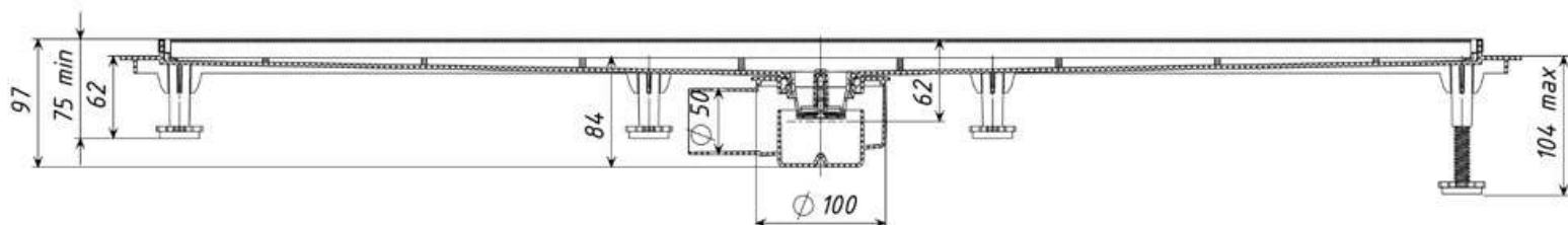
Вариант установки механического "сухого" затвора
