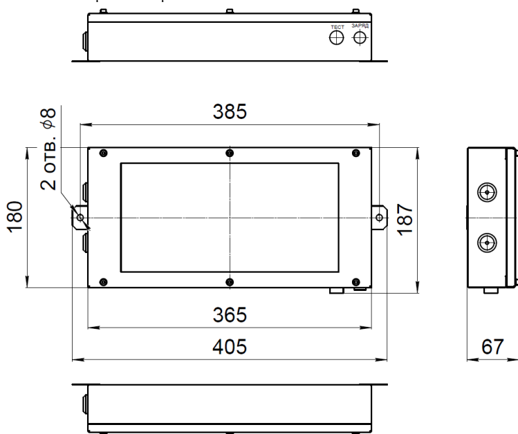
Рис. №3 Габаритный чертёж.
