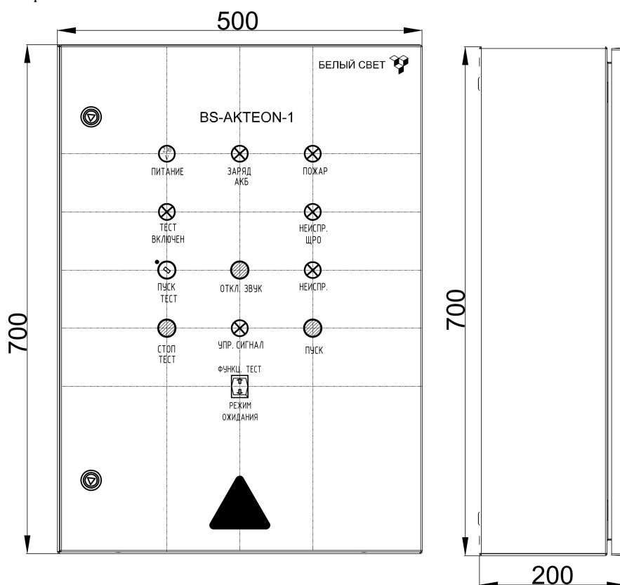
Рис. №1 Габаритный чертёж.
