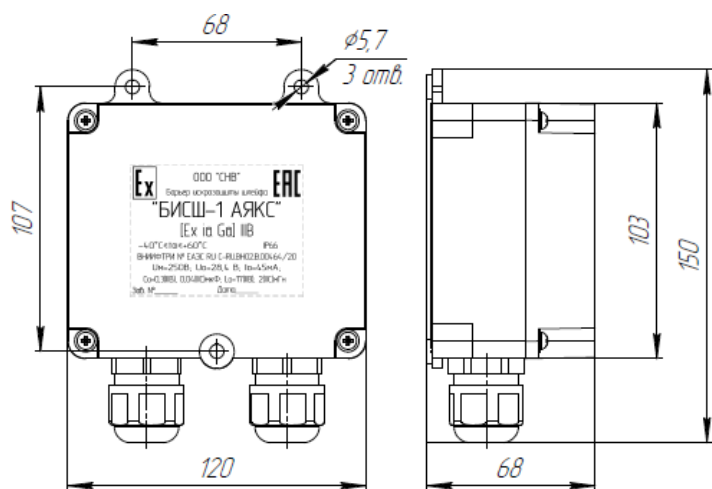
БИСШ-1 АЯКС,
