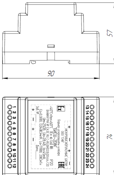
БИСШ-2DIN АЯКС
