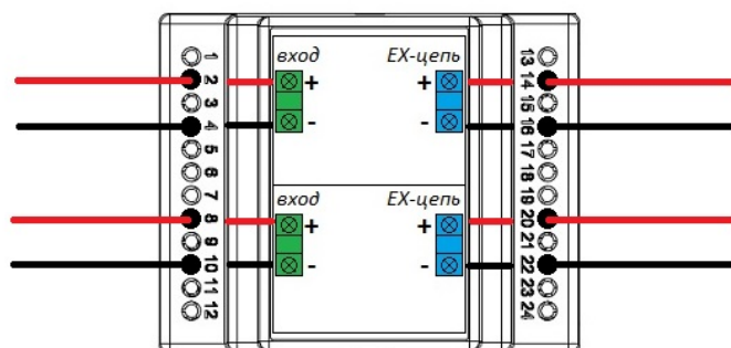
БИСШ-2 АЯКС
