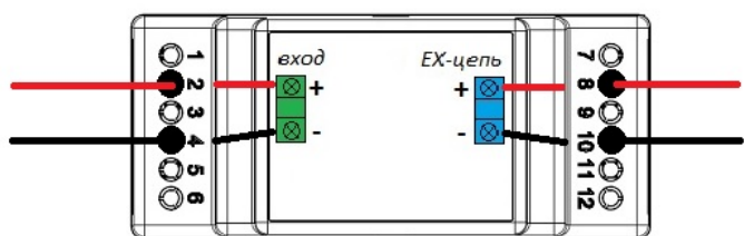
схемы подключения БИСШ-1DIN АЯКС, БИСШ-2DIN АЯКС
