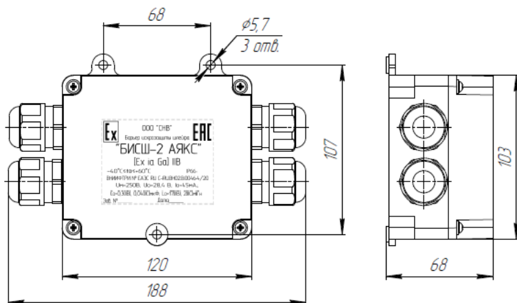
БИСШ-2 АЯКС
