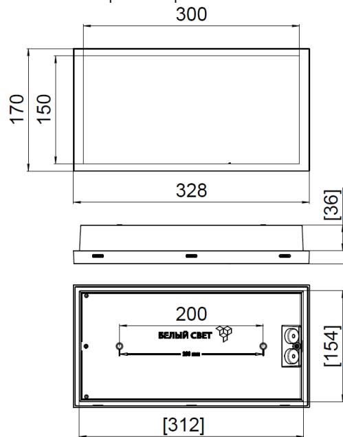
Рис. №2 Габаритный чертёж.
