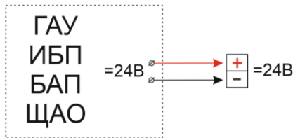
Приложение № 2. Схемы подключения, габаритные чертежи и аксессуары. Рис. №1 Схема подключения к групповой цепи питания.
