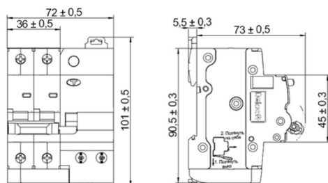
Рис. 6. Габаритные и установочные размеры УЗДП 25-63 А
