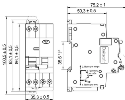
Рис. 5. Установочные и габаритные размеры УЗДП 10-20 А
