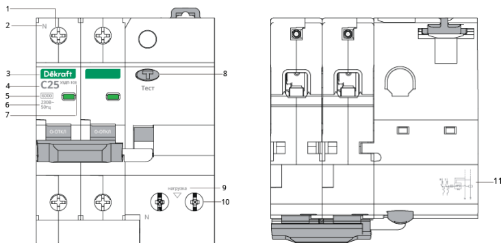
Рис. 2. Внешний вид УЗДП 25-63 А
