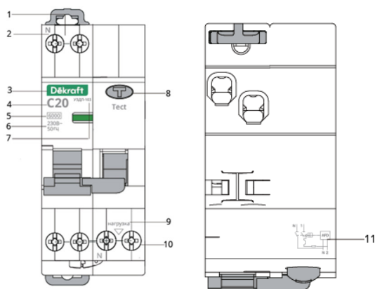
Рис. 1. Внешний вид УЗДП 10–20 А
