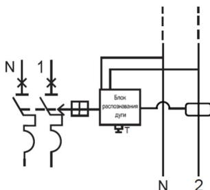
Рис. 3. Схема функциональная УЗДП
