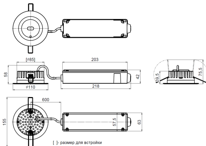
Рис. №2 Габаритный чертёж. BS-ARUNA-81-L1-INEXI3 IP65 BS-ARUNA-81-L2-INEXI3 IP65 BS-ARUNA-81-L3-INEXI3 IP65
