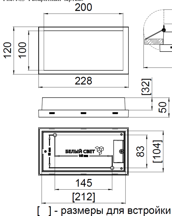
Рис. №3 Габаритный чертёж.
