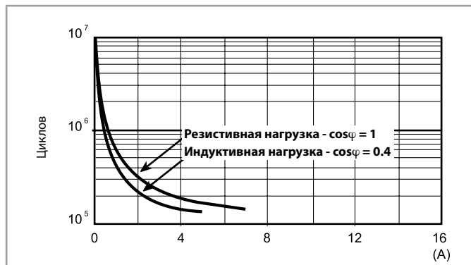
F 58 - Электрическая долговечность (АС) при ном. нагрузке Реле с 4 перекидными контактами
