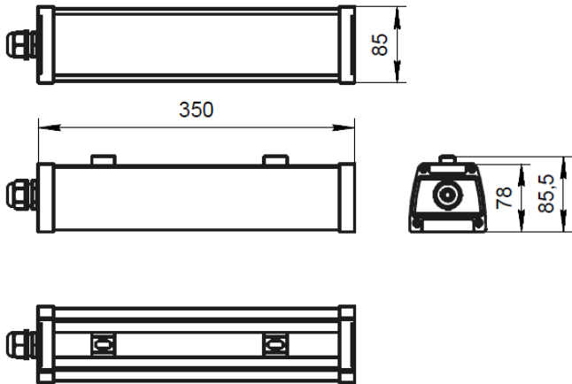
Рис. №2 Габаритный чертёж.
