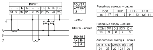
ф) схема подключения мультиметра LED к трехпроводной сети при I > 5 \text{ A} , U > 600 \text{ В}
