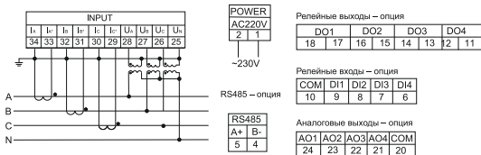
е) схема подключения мультиметра LED к четырехпроводной сети при I > 5 \text{ A} , U > 600 \text{ В}
