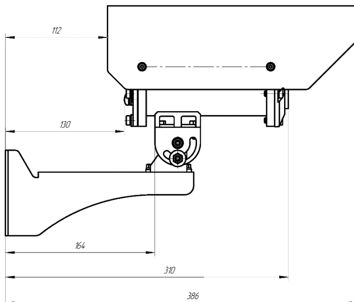
Рисунок А2. Габаритные размеры Спектрон-801-Exd-M/H-HART
