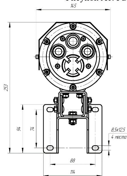
Рисунок А1. Габаритные размеры Спектрон-801-Exd-A-HART
