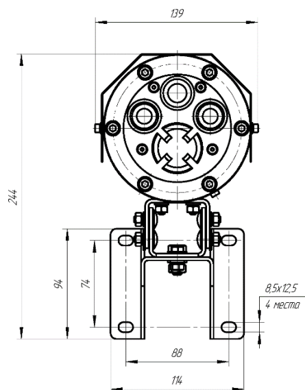
Рисунок А1. Габаритные размеры Спектрон-801-Exd-A-HART
