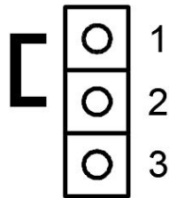
Рисунок 10 – Установка джампера согласующего резистора Переключатель в положении «1-2» – согласующий резистор подключен . Переключатель в положении «2-3» – согласующий резистор отключен .
