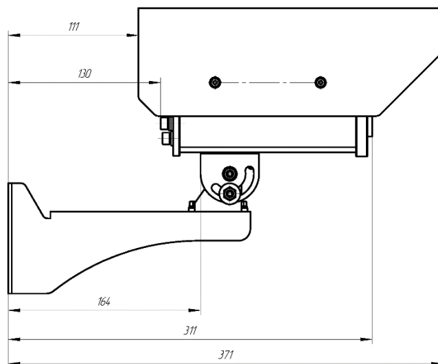
Рисунок А1. Габаритные размеры Спектрон-801-Exd-A-HART
