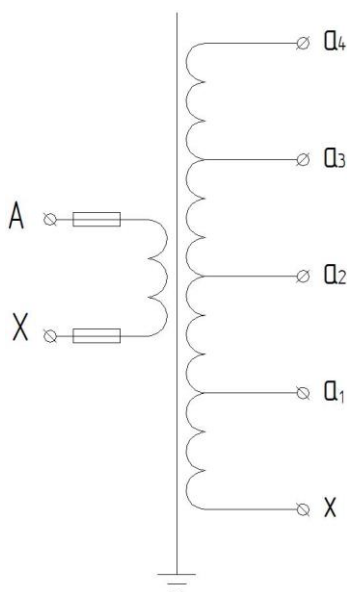
Рисунок Б.2 – Схема электрическая принципиальная трансформаторов ОЛСП-НТЗ-0,63/6(10), ОЛСП-НТЗ-1,25/6(10)
