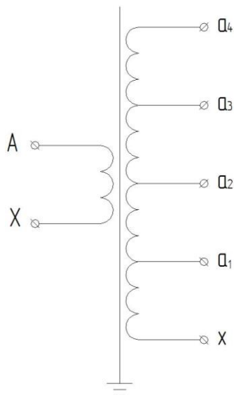
Рисунок Б.1 – Схема электрическая принципиальная трансформаторов ОЛС-НТЗ-0,63/6(10), ОЛС-НТЗ-1,25/6(10)
