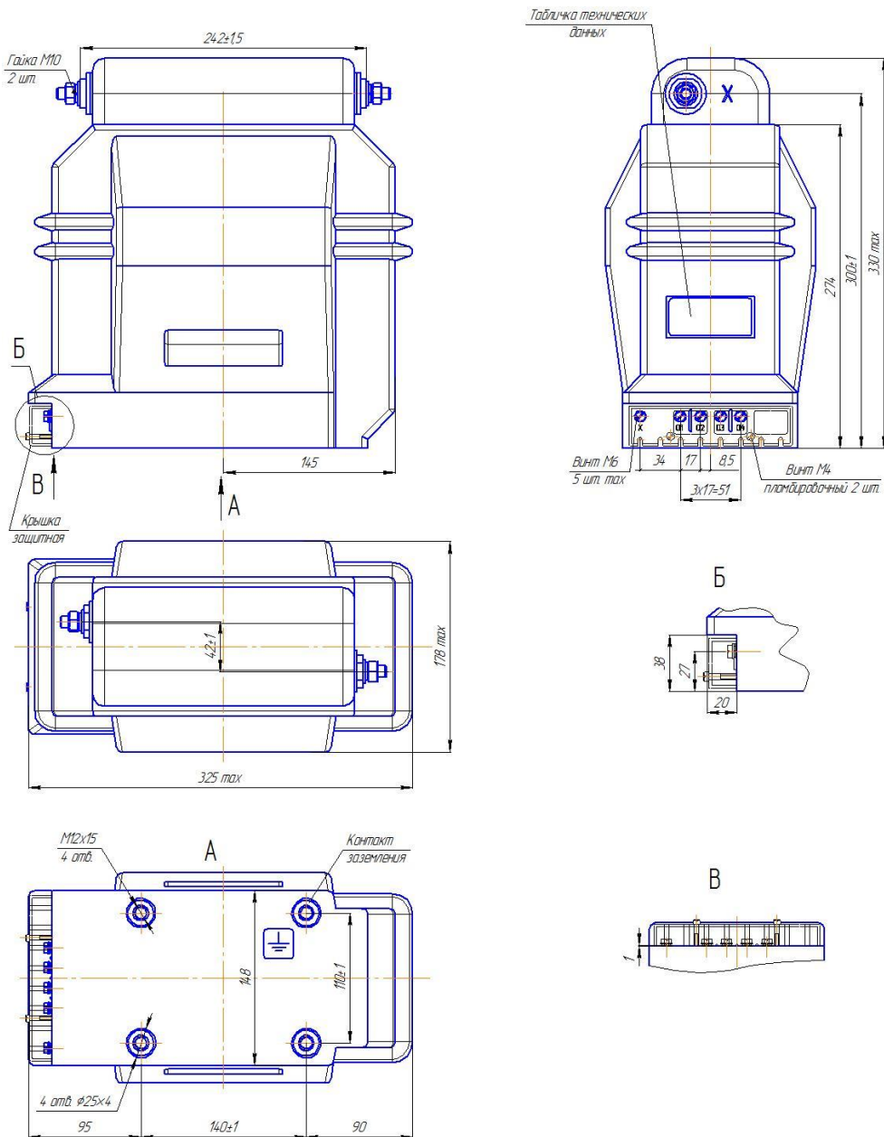
Рисунок А.4 – Габаритные, установочные, присоединительные размеры и масса трансформатора ОЛСП-НТЗ-1,25/6(10)
