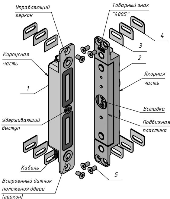
Рисунок 1- Комплект поставки
