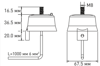
Габаритные и установочные размеры
