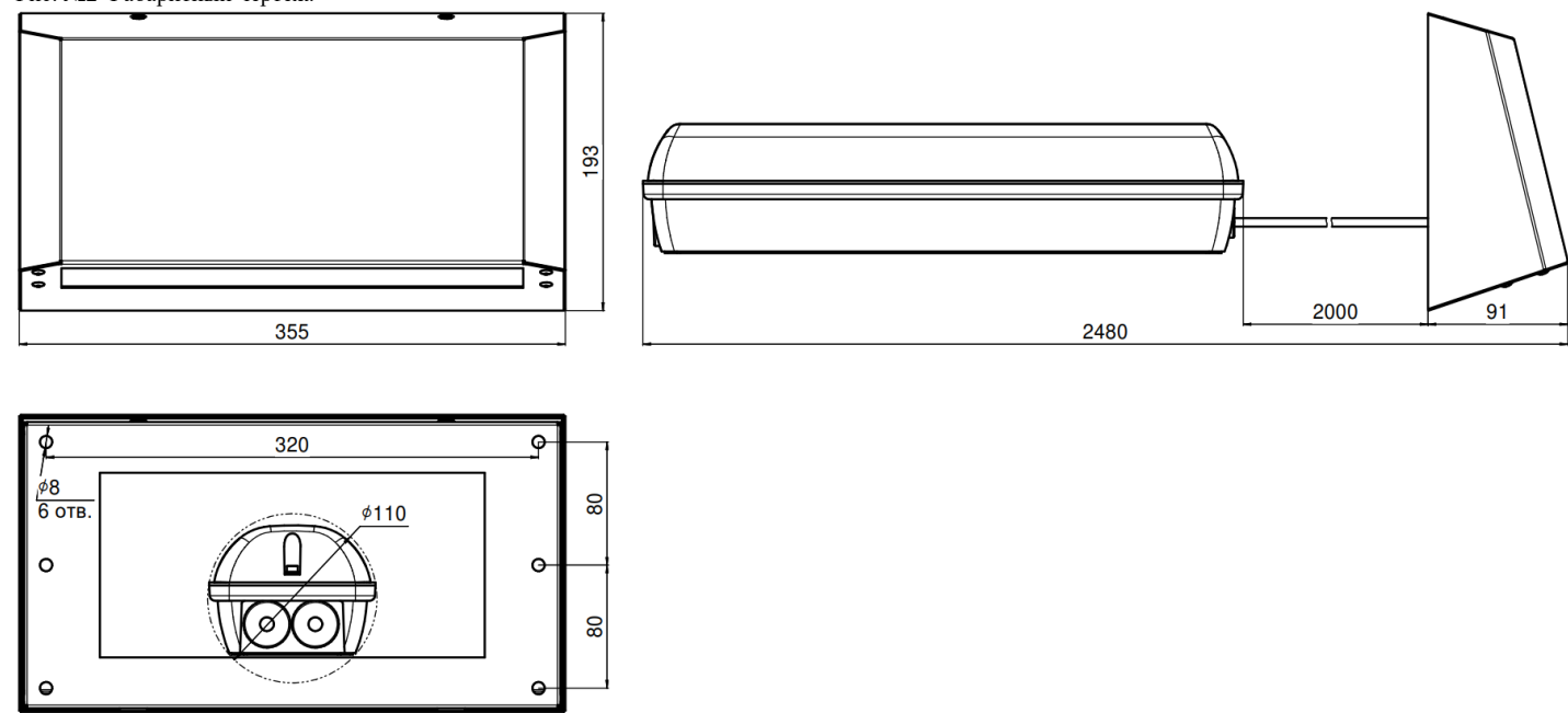
Рис. №2 Габаритный чертёж.
