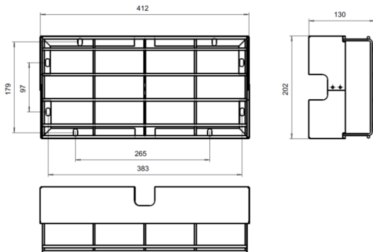
Рис. №6 Аксессуары. Решётка защитная BS-R-1 (a2333)
