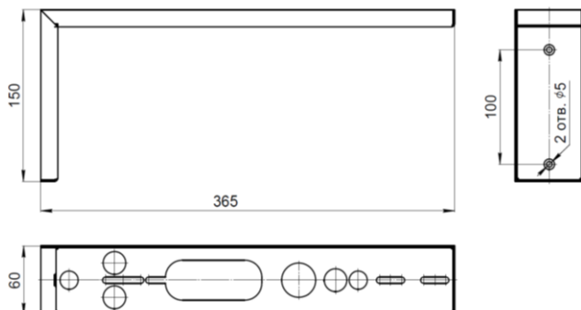
Рис. №7 Кронштейн BS-K-3
