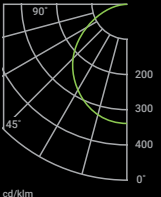
Опал 40 Вт
