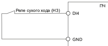
Рисунок В.7 – Схема подключения защиты от «сухого» хода (Н3)
