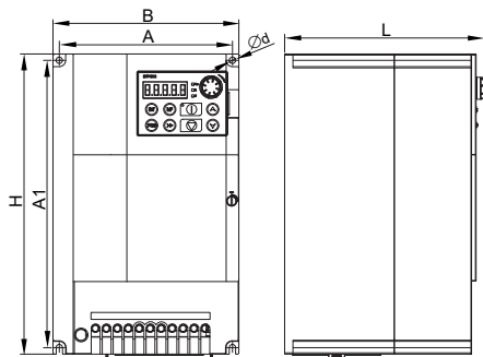
Рисунок 2.3 – Габаритные и установочные размеры преобразователя (габариты 3-4)
