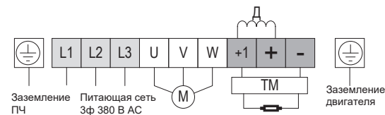
г) преобразователь мощностью 30 – 37 кВт
