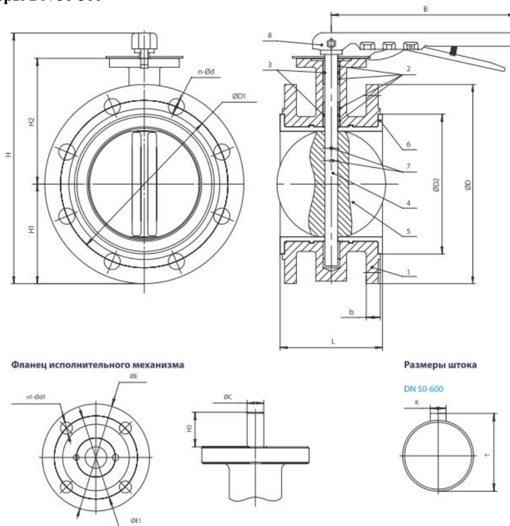
Рисунок 1. Затворы DN 50-300
