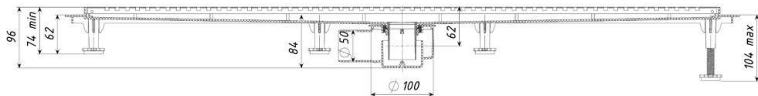
Вариант установки с гидрозатвором
