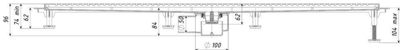
Вариант установки механического "сухого" затвора
