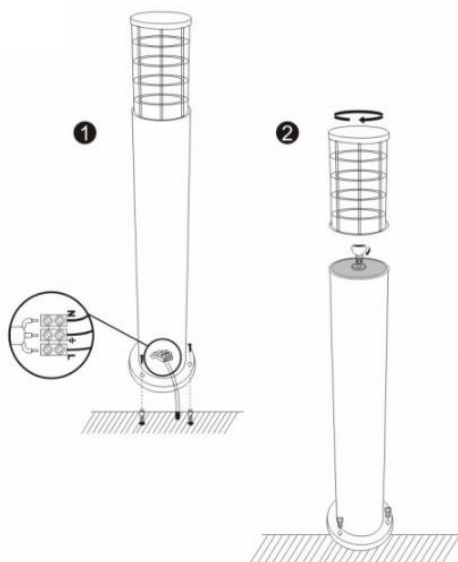
Рис. 1 Внешний вид светильника
