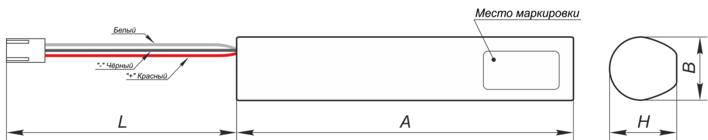
Рис.8 Габаритный чертеж Батареи
